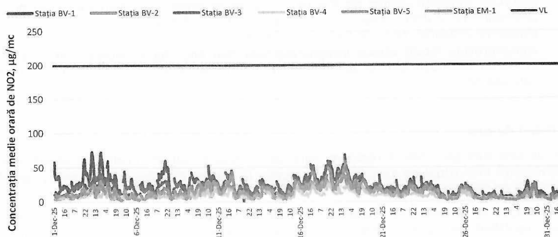
Figura 3. Concentrații medii orare de NO 2 în luna decembrie 2025
