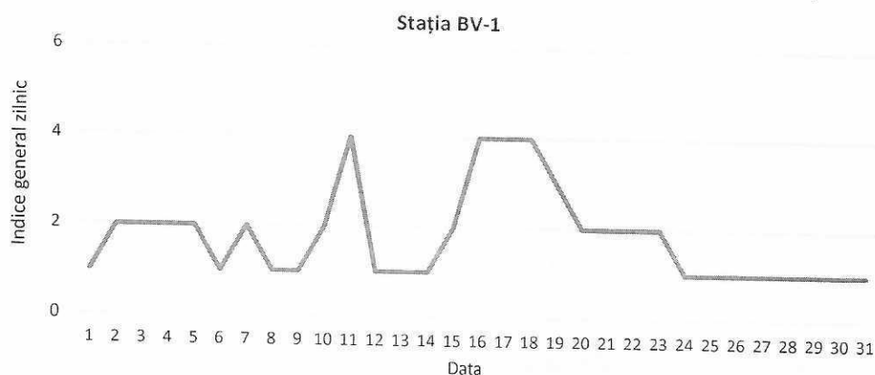
Figura 16. Evoluția indicelui general de calitatea aerului din stația BV-1
