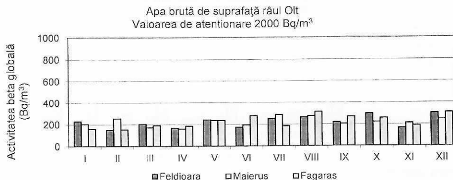
Fig. 29. Activitatea beta globală la 5 zile pentru apa de suprafață Râul Olt
