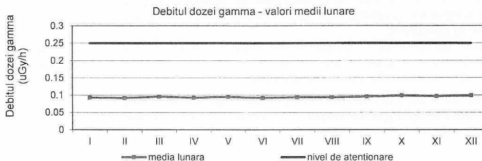
Figura 25. Debitul dozei gamma
