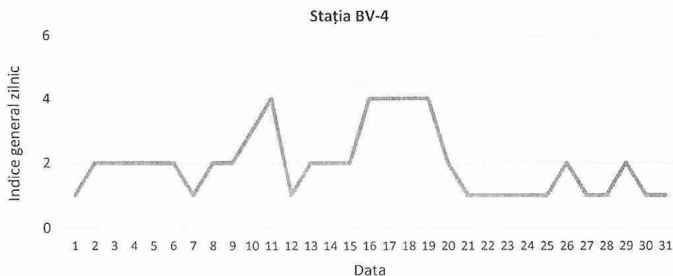
Figura 19. Evoluția indicelui general de calitate a aerului din stația BV-4
