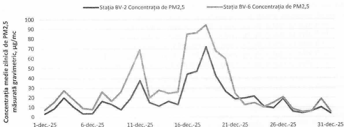
Figura 13. Evoluția concentrațiilor medii zilnice de PM 2,5 (gravimetric) în luna decembrie 2025
