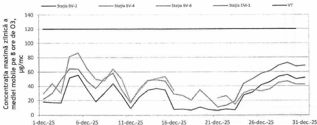
Figura 5. Evoluția concentrațiilor maximelor zilnice ale mediilor mobile pe 8 ore de O 3 în luna decembrie 2025
