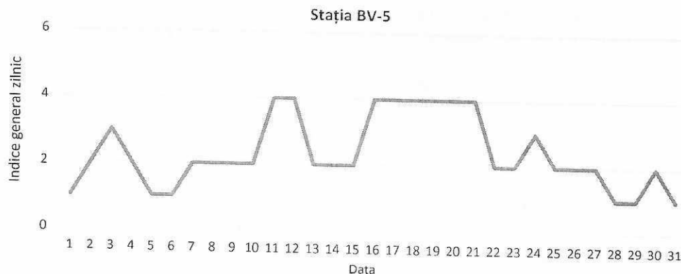
Figura 20. Evoluția indicelui general de calitate a aerului din stația BV-5
