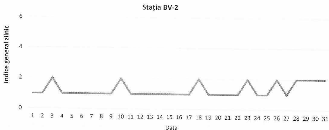
Figura 17. Evoluția indicelui general de calitatea aerului din stația BV-2
