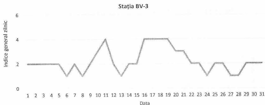
Figura 18. Evoluția indicelui general de calitate a aerului din stația BV-3
