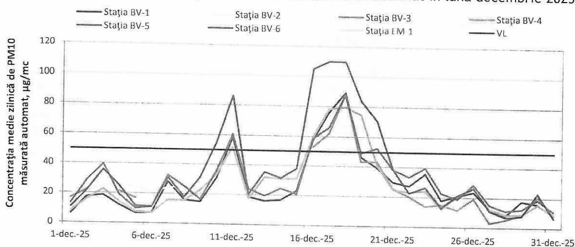
Figura 12. Evoluția concentrațiilor medii zilnice de PM 10 automat în luna decembrie 2025
