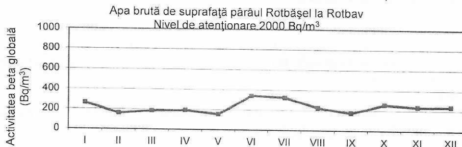
Figura 28. Activitatea beta globală la 5 zile pentru apa de suprafață-Pârâul Rotbășel
