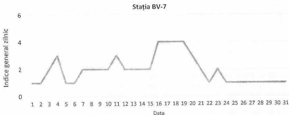
Figura 22. Evoluția indicelui general de calitate a aerului din stația BV-7
