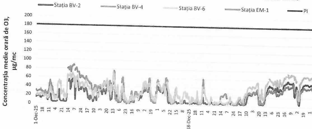
Figura 6. Evoluția concentrațiilor medii orare de O 3 în luna decembrie 2025
