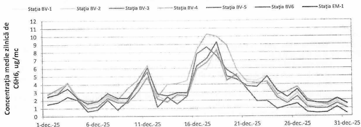
Figura 7. Evoluția concentrațiilor medii zilnice de benzen în luna decembrie 2025
