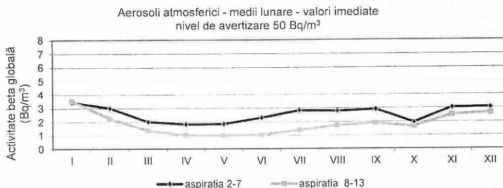
Figura 23. Activitatea beta globală pentru aerosoli atmosferici
