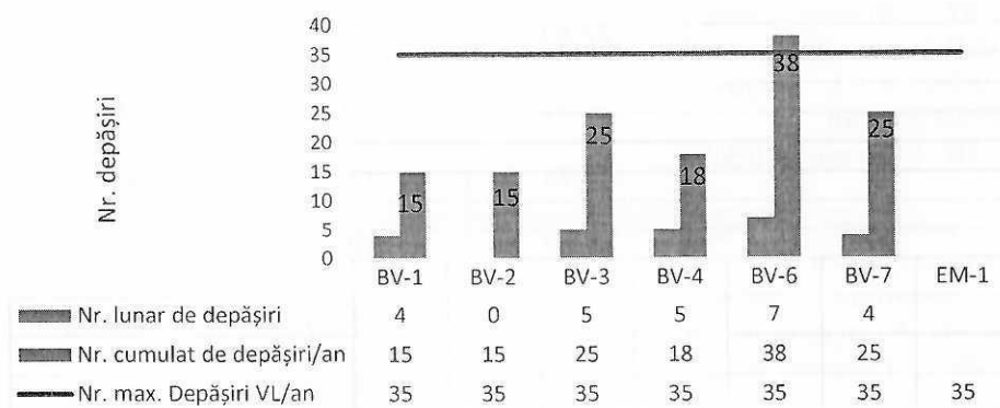
Figura 11. Numărul lunar și cumulat de depășiri ale valorii limită zilnice la PM10
