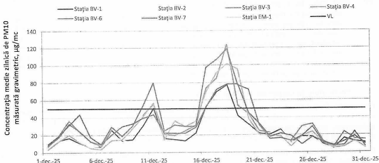
Figura 10. Evoluția concentrațiilor medii zilnice de PM10 (gravimetric) în luna decembrie 2025
