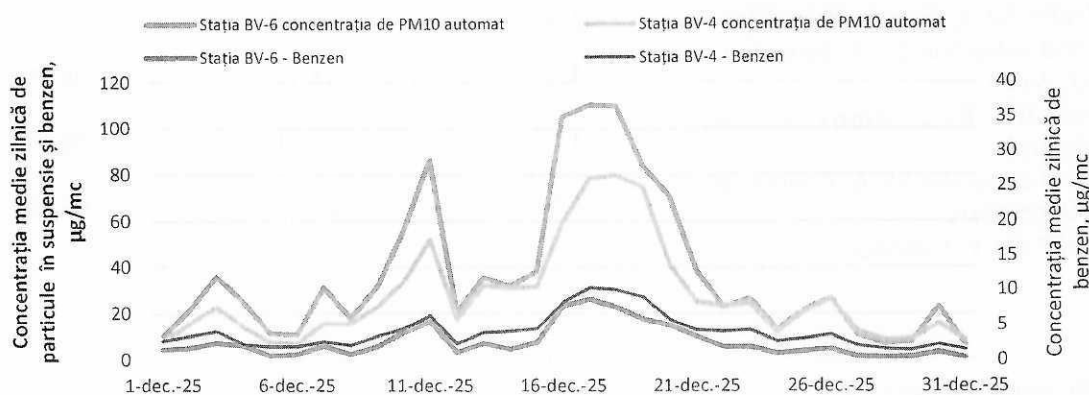
Figura 9. Evoluția concentrațiilor medii zilnice de benzen și particule în suspensie în luna decembrie 2025
