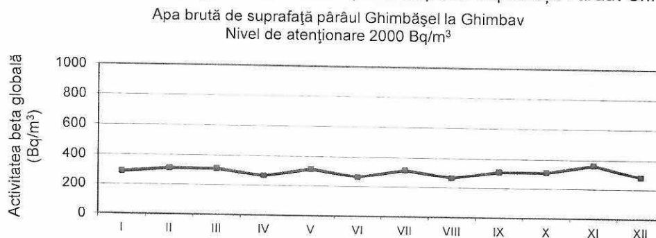
Figura 27. Activitatea beta globală imediată pentru apa de suprafață Pârâul Ghimbășel
