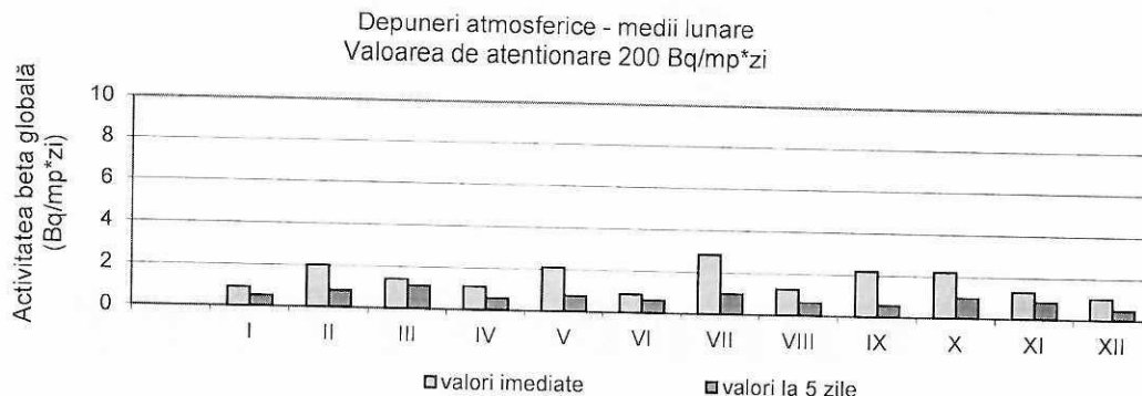
Figura 26. Activitatea beta globală pentru depuneri atmosferice
